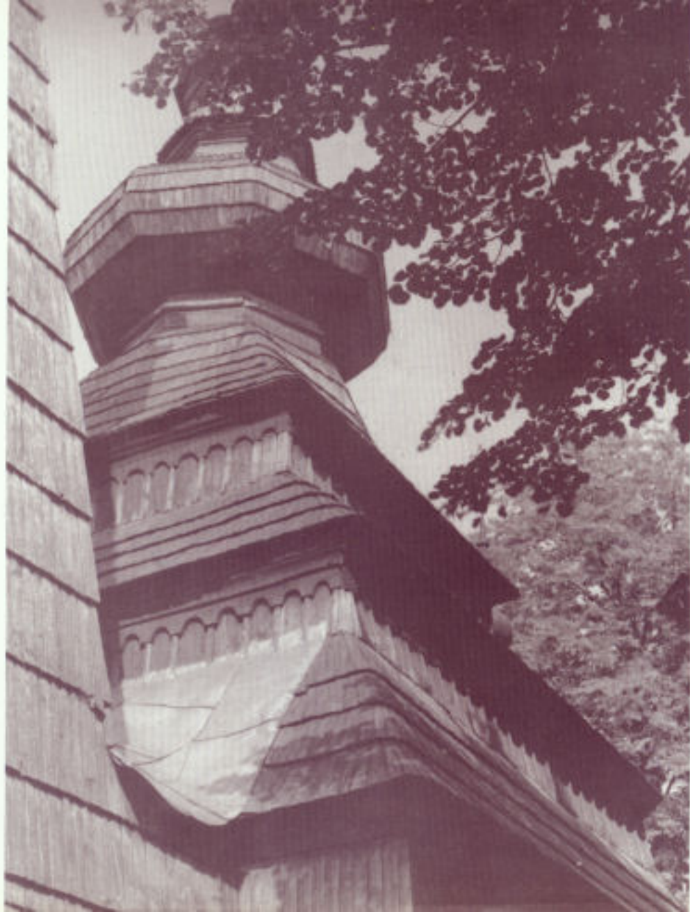
121. Kwiatotł, Polska. Cerkiew gr.-kat.; fragment zadaszeń kopuły nawy i wieńczącej ją wieżyczki; zapewne 2. poł. w. XVII. Widok od pd.-zach.
